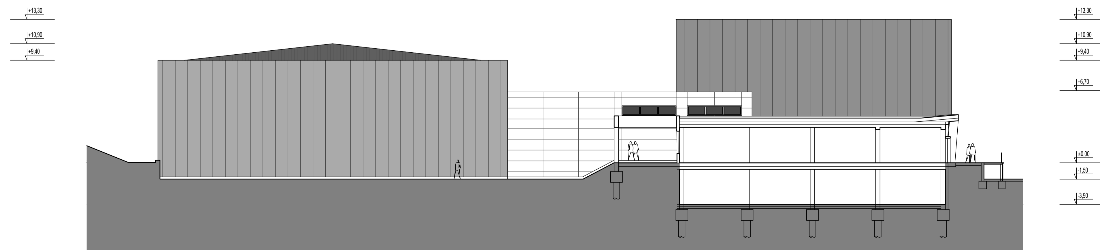
řezopohled východní
