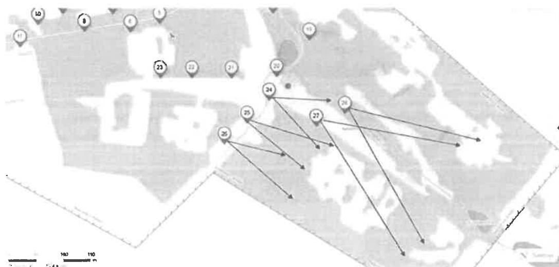
Rozmístění střeleckých stanovišť č.24 až 28, a jejich střeleckých výsečí (primárních ohrožených prostorů pro každé střelecké stanoviště).
